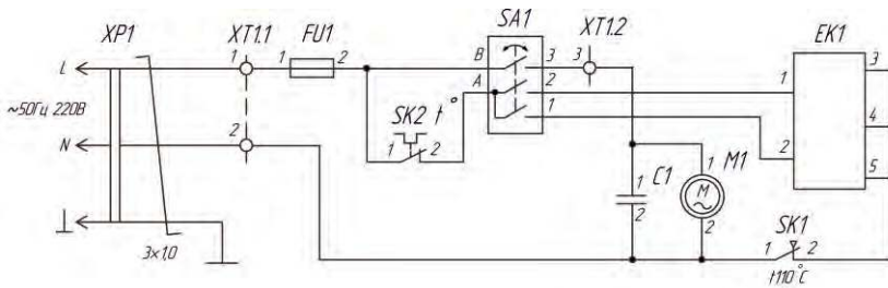
Схема коммутации переключателя SA1
