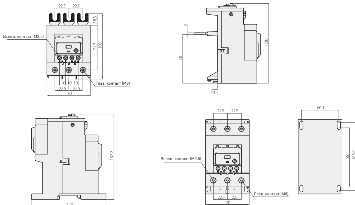
HGT100
