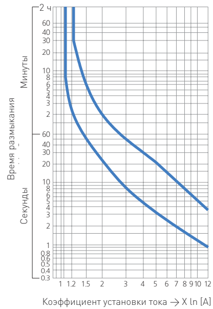
HGT40K
