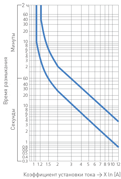
HGT400K
