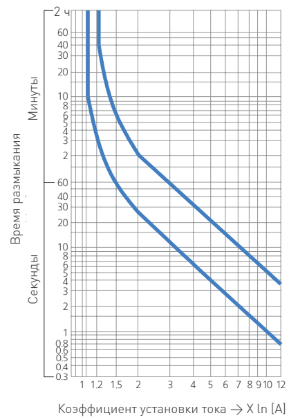
HGT265K
